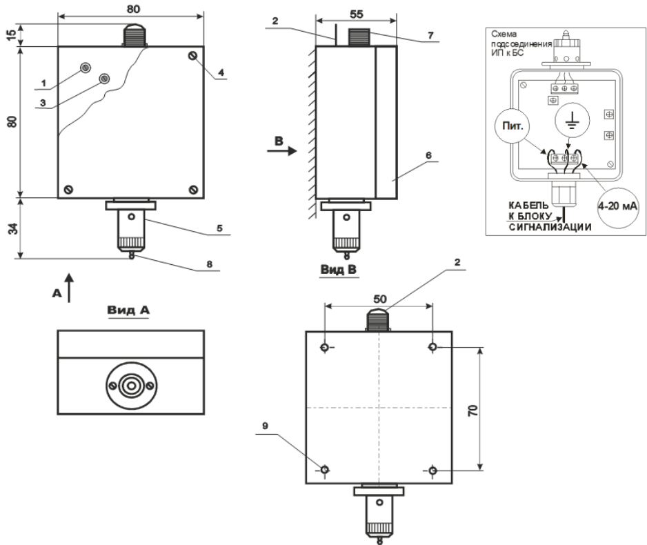
РИС.46. ИП МН-2,5. Габаритные и установочные размеры
