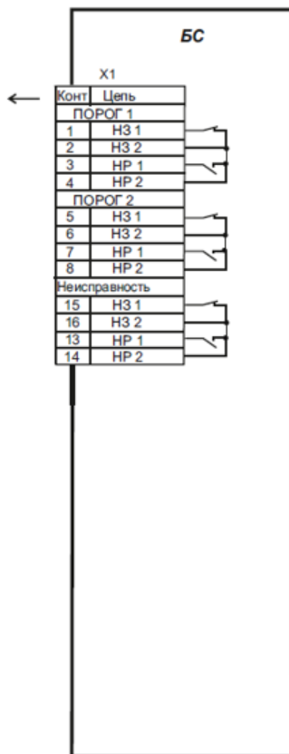
РИС. 7. Схема выходных разъемов БС для связи с внешними исполнительными устройствами X1 – разъем для подключения внешних устройств, вилка 2PM24KPN19Ш1В
